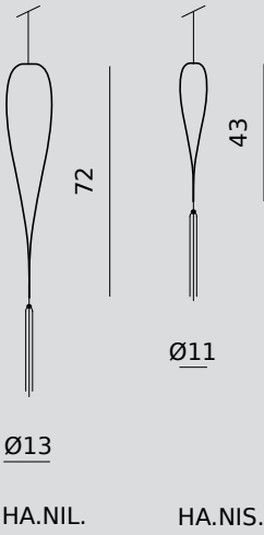
LAMPADA A SOSPENSIONE IN VETRO SOFFIATO RIGATO TRASPARENTE O SATINATO, CON PASSAMANERIA LUNGH. 40 CM INCLUSA. UTILIZZABILE ANCHE CON SUPPORTI DA PARETE E DA TERRA. HANGING LAMP, RULED HAND BLOWN GLASS TRANSPARENT OR FROSTED WITH 40 CM. LENGHT TASSEL INCLUDED. ALSO AVAILABLE WITH WALL AND FLOOR SUPPORT.
