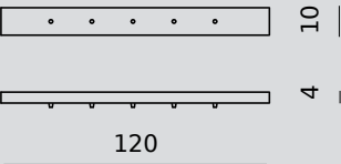
CIELINO RETTANGOLARE 5 LAMPADE RECTANGULAR CEILING 5 LAMPS SU.R5
